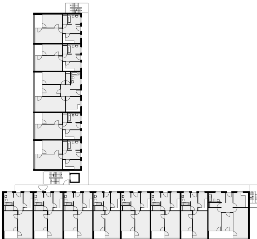
2. OBERGESCHOSS
